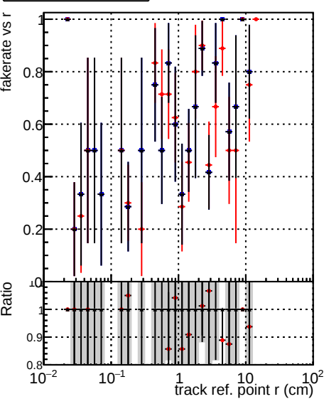
Fake rate vs DOM CKFFit 1000evt DOM CKFREFit 1000evt DOM NOTESTCKF 1000evt
