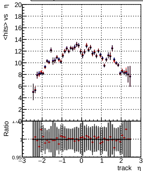
mean hits vs \eta — DQM_CKFFit_1000evt — DQM_CKFREFit_1000evt — DQM_NOTESTCKF_1000evt
