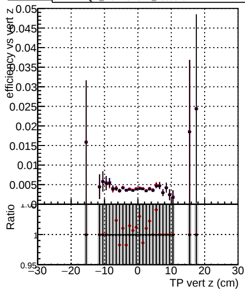
Efficiency vs vert z — DQM_CKFFit_1000evt — DQM_CKFFit_1000evt — DQM_NOTESTCKF_1000evt
