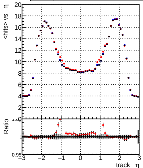
mean hits vs \eta — DQM_CKFFit_1000evt — DQM_CKFREFit_1000evt — DQM_NOTESTCKF_1000evt
