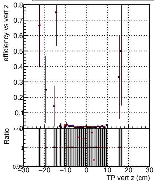
Efficiency — DQM_CKFFit_1000evt — DQM_CKFFit_1000evt — DQM_NOTESTCKF_1000evt
