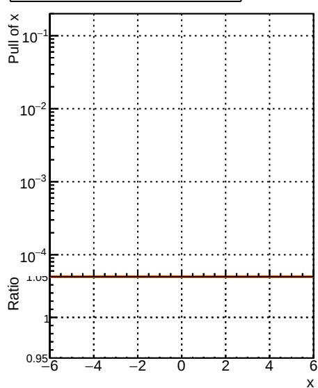
RecoAllAssoc2GenMatched_PulIX
