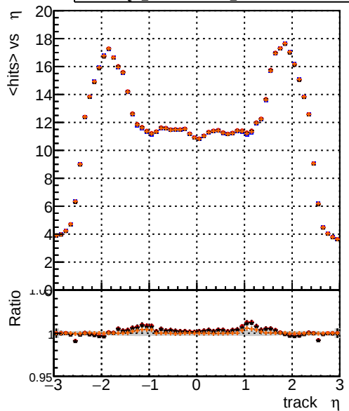
mean hits vs \eta DOM_CKFFit_1000evt DOM_CKFREFit_1000evt DOM_NANTESTCKF2_1000evt DOM_NANTESTCKF3_1000evt
