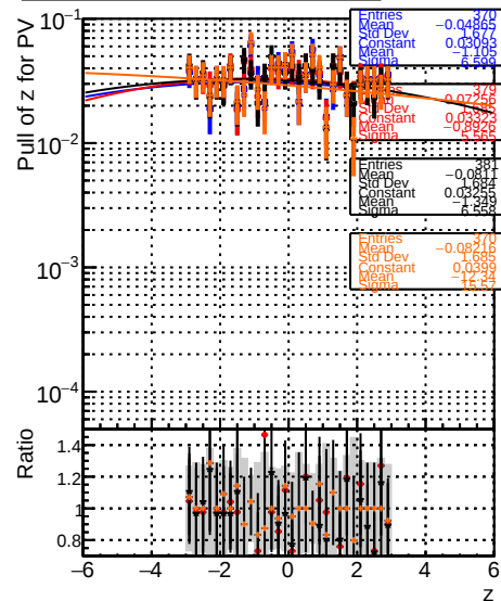
RecoPVAssoc2GenPVMatched_PulIZ
