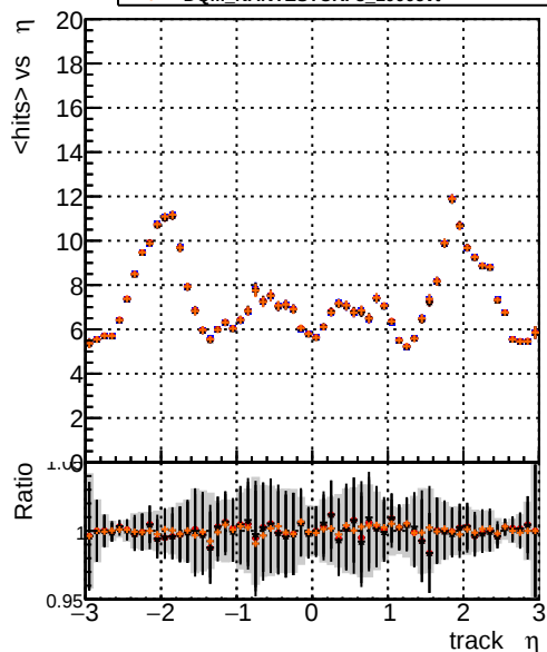
mean hits vs \eta DOM_CKFFit_1000evt DOM_CKFREFit_1000evt DOM_NANTESTCKF2_1000evt DOM_NANTESTCKF3_1000evt
