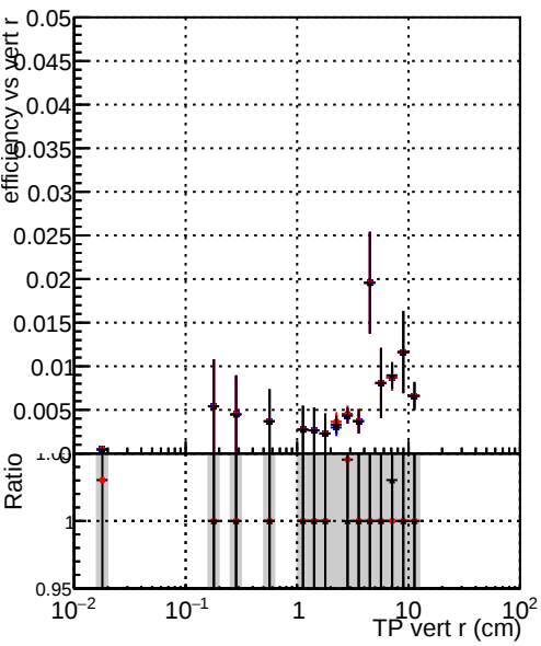
Efficiency vs vertpos DQM_CKF-testLowPt_1000evt DQM_CKFREFit-testLowPt_1000evt DQM_mkFitREFit-testLowPt_1000evt
