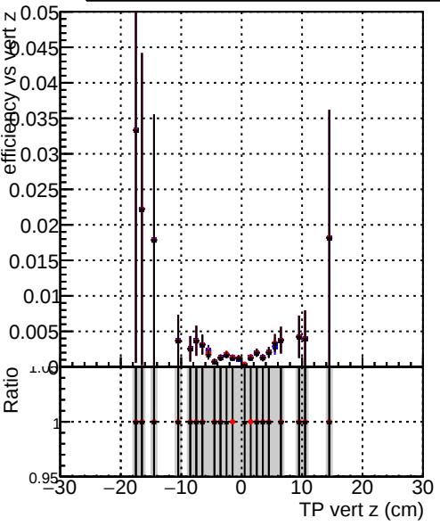
Efficiency vs vertpos Legend: DQM_CKF-testLowPt_1000evt DQM_CKFREFit-testLowPt_1000evt DQM_mkFitREFit-testLowPt_1000evt
