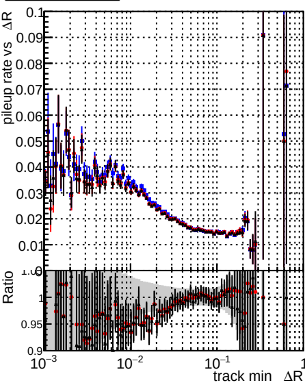
Legend: DQM_CKF-testLowPt_1000evt (blue squares), DQM_CKFREFit-testLowPt_1000evt (red circles), DQM_mkFitREFit-testLowPt_1000evt (black triangles)
