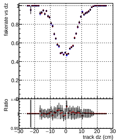
Fake rate vs dz DOM CKE testLowPt_1000evt DOM CKF testLowPt_1000evt DOM CKF REFit testLowPt_1000evt
