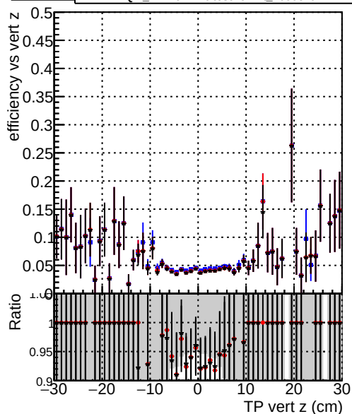
Efficiency vs vert z —•— DQM_CKF-testLowPt_1000evt —•— DQM_CKFREFit-testLowPt_1000evt —•— DQM_mkFitREFit-testLowPt_1000evt
