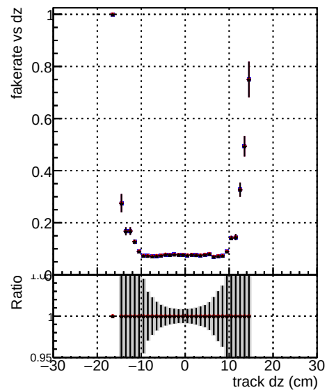
Fake rate vs dz DOM CKE testLowPt_1000evt DOM CKE testLowPt_1000evt DOM mktFit-testLowPt_1000evt
