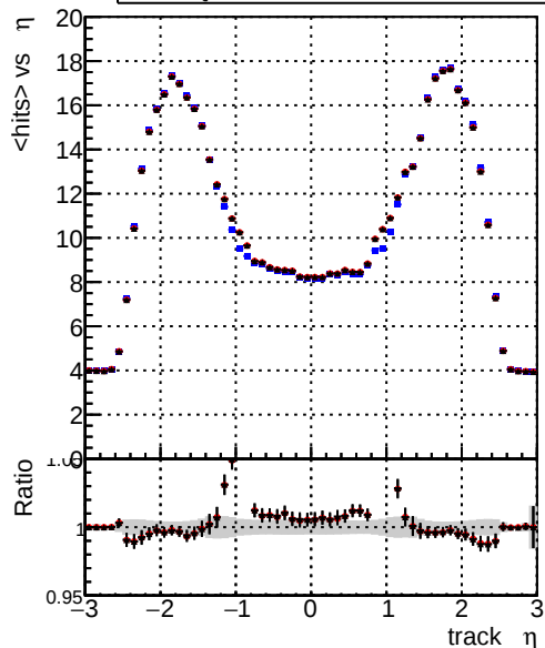
mean hits vs \eta — DQM_CKF-testLowPt_1000evt — DQM_CKFREFit-testLowPt_1000evt — DQM_mkFitREFit-testLowPt_1000evt
