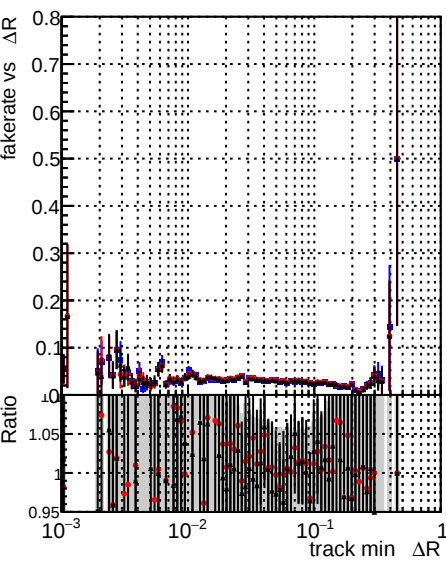
Fake rate vs \Delta R(\text{track, jet}) Legend: DQM_CKF-testLowPt_1000evt DQM_CKFREFit-testLowPt_1000evt DQM_mkFitREFit-testLowPt_1000evt
