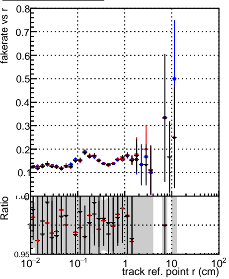
Fake rate vs —■— DQM_CKF-testLowPt_1000evt —●— DQM_CKFREFit-testLowPt_1000evt —▲— DQM_mkFitREFit-testLowPt_1000evt
