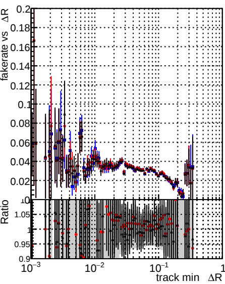
—■— DOM_CKF-testLowPt_1000evt —●— DOM_CKFREFit-testLowPt_1000evt —×— DOM_mkFitREFit-testLowPt_1000evt
