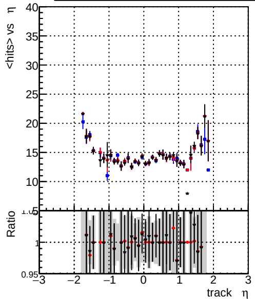
mean hits vs \eta — DQM_CKF-testLowPt_1000evt — DQM_CKFREFit-testLowPt_1000evt — DQM_mkFitREFit-testLowPt_1000evt
