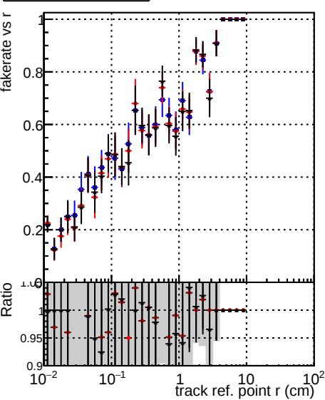
Fake rate vs DOM_CKF-testLowPt_1000evt DOM_CKFREFit-testLowPt_1000evt DOM_mkFitREFit-testLowPt_1000evt
