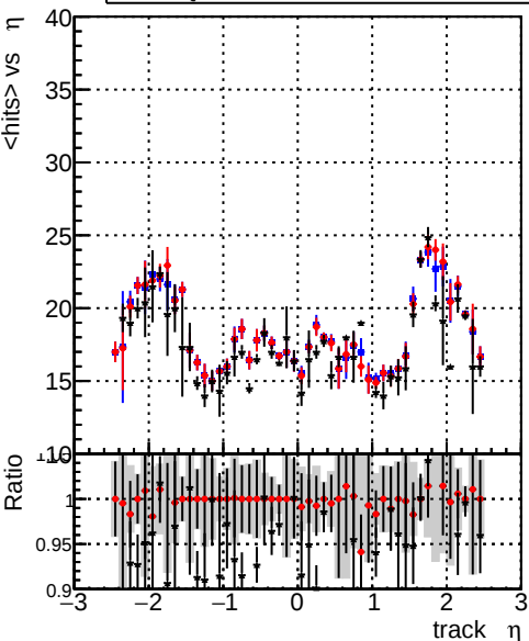
mean hits vs \eta DQM_CKF-testLowPt_1000evt DQM_CKFREFit-testLowPt_1000evt DQM_mkFitREFit-testLowPt_1000evt
