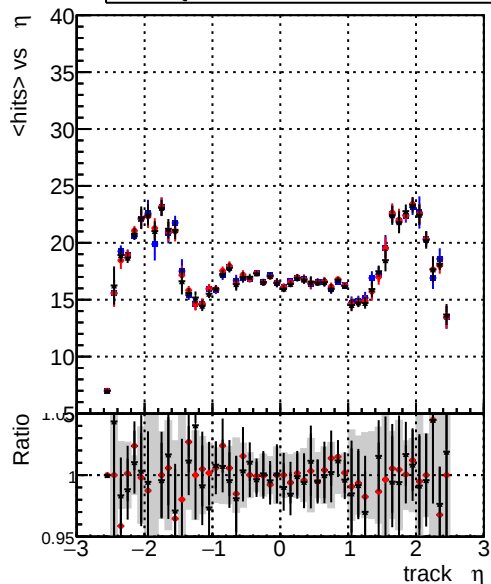
mean hits vs \eta — DQM_CKF-testLowPt_1000evt — DQM_CKFFit-testLowPt_1000evt — DQM_mkFitREFit-testLowPt_1000evt
