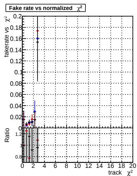
Fake rate vs. DOM CKF testLowPt 1000evt DOM CKF testLowPt 1000evt DOM CKF testLowPt 1000evt
