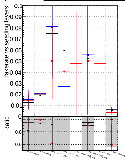
Fake rate vs. DOM CKF testLowPt 1000evt DOM CKF testLowPt 1000evt DOM CKF testLowPt 1000evt
