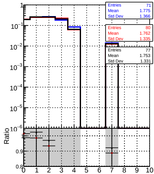
mean hits vs \eta — DQM_CKF-testLowPt_1000evt — DQM_CKFFit-testLowPt_1000evt — DQM_mkFitREFit-testLowPt_1000evt
