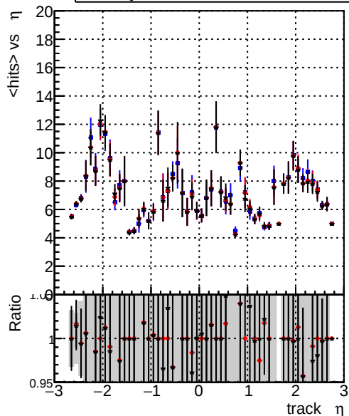
mean hit — DQM_CKF-testLowPt_1000evt — DQM_CKFREFit-testLowPt_1000evt — DQM_mkFitREFit-testLowPt_1000evt
