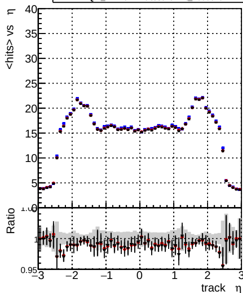
mean hits — DQM_CKF-testLowPt_1000evt — DQM_CKFREFit-testLowPt_1000evt — DQM_mkFitREFit-testLowPt_1000evt
