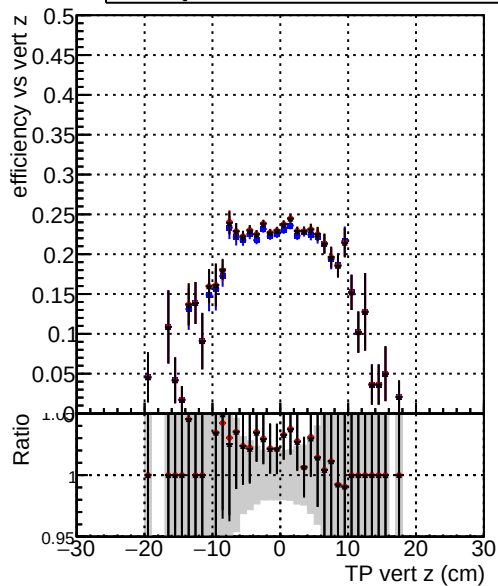
Efficiency vs vert z —•— DQM_CKF-testLowPt_1000evt —•— DQM_CKFFit-testLowPt_1000evt —•— DQM_mkFitREFit-testLowPt_1000evt
