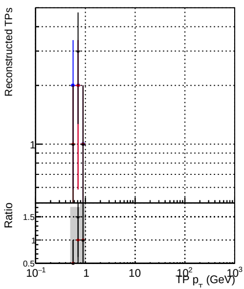
—•— DQM_CKF-testLowPt_1000evt —•— DQM_CKFFit-testLowPt_1000evt —•— DQM_mkFitREFit-testLowPt_1000evt
