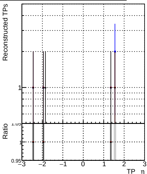
—•— DQM_CKF-testLowPt_1000evt —•— DQM_CKFFit-testLowPt_1000evt —•— DQM_mkFitREFit-testLowPt_1000evt
