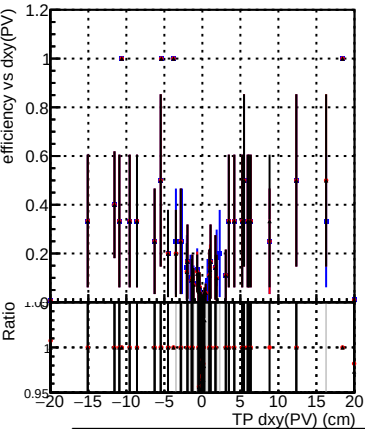
Efficiency vs Dxy(PV) Legend: DQM_CKF-testLowPt_1000evt DQM_CKFREFit-testLowPt_1000evt DQM_mkFitREFit-testLowPt_1000evt
