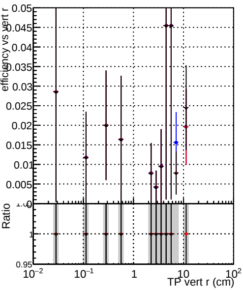
Efficiency vs vertpos DQM_CKF-testLowPt_1000evt DQM_CKFFit-testLowPt_1000evt DQM_mkFitREFit-testLowPt_1000evt
