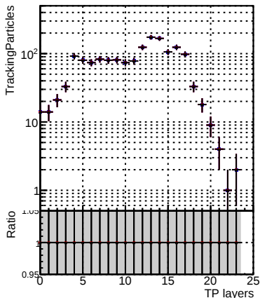
N of sim \rightarrow DQM_mkFitREFit-
