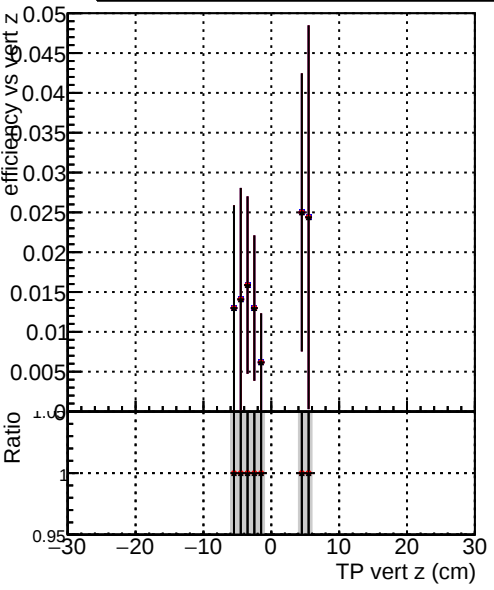
Efficiency vs vertpos Legend: DQM_CKF-testLowPt_1000evt DQM_CKFFit-testLowPt_1000evt DQM_mkFitREFit-testLowPt_1000evt
