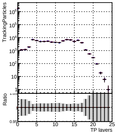
N of sim \rightarrow DQM_mkFitREFit-testLowPt_1000evt
