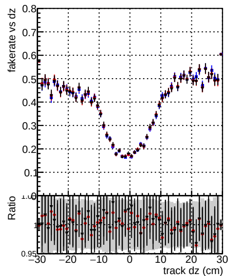
Fake rate vs dz Legend: DOM CKF-testLowPt_1000evt DOM CKF-testLowPt_1000evt DOM CKF-testLowPt_1000evt
