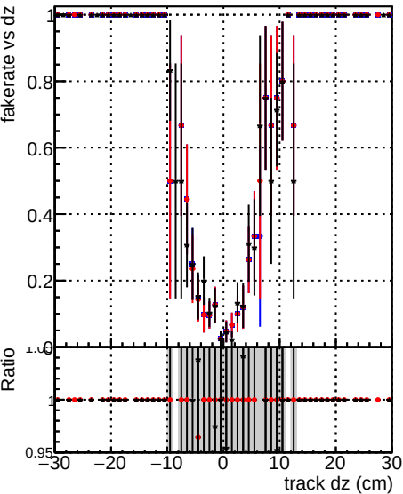
Fake rate vs dz DOM CKE testLowPt_1000evt DOM CKE testLowPt_1000evt DOM mkr testLowPt_1000evt
