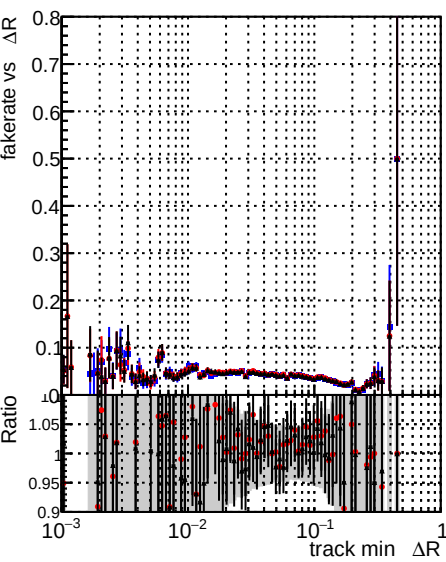
Fake rate vs \Delta R(\text{track}, \text{jet}) Legend: DOM CKFit-testLowPt 1000evt DOM CKFitREFit-testLowPt 1000evt DOM mkFitREFit-testLowPt 1000evt
