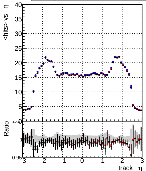
mean hits — DQM_CKF-testLowPt_1000evt — DQM_CKFREFit-testLowPt_1000evt — DQM_mkFitREFit-testLowPt_1000evt
