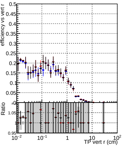
Efficiency vs vertpos Legend: DQM_CKF-test_1000evt DQM_CKFitFit-test_1000evt DQM_mkFitFit-test_1000evt
