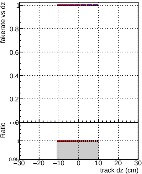
Fake rate vs dz DOM CKE test 1000evt DOM CKE fit test 1000evt DOM mkr fit test 1000evt
