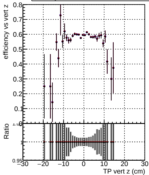
Efficiency vs. TP vert z — DQM_CKF-test_1000evt — DQM_CKFREFit-test_1000evt — DQM_mkFitREFit-test_1000evt
