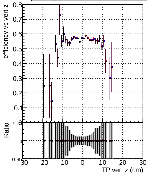
Efficiency vs vert z —●— DQM_CKF-test_1000evt —●— DQM_CKFREFit-test_1000evt —●— DQM_mkFitREFit-test_1000evt
