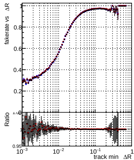
—•— DOM CKFit-test 1000evt —•— DOM CKFitREFit-test 1000evt —•— DOM mkFitREFit-test 1000evt
