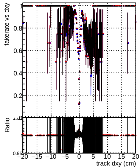
— DOM CKF test 1000evt — DOM CKF test 1000evt — DOM CKF test 1000evt
