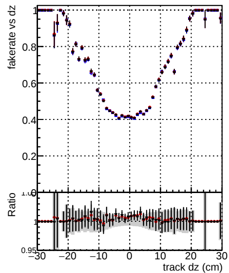
— DOM CKF test 1000evt — DOM CKF test 1000evt — DOM CKF test 1000evt
