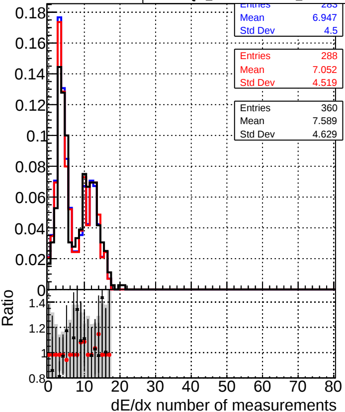
— DQM_CKF-test_1000evt — DQM_CKFREFit-test_1000evt — DQM_mkFitREFit-test_1000evt
