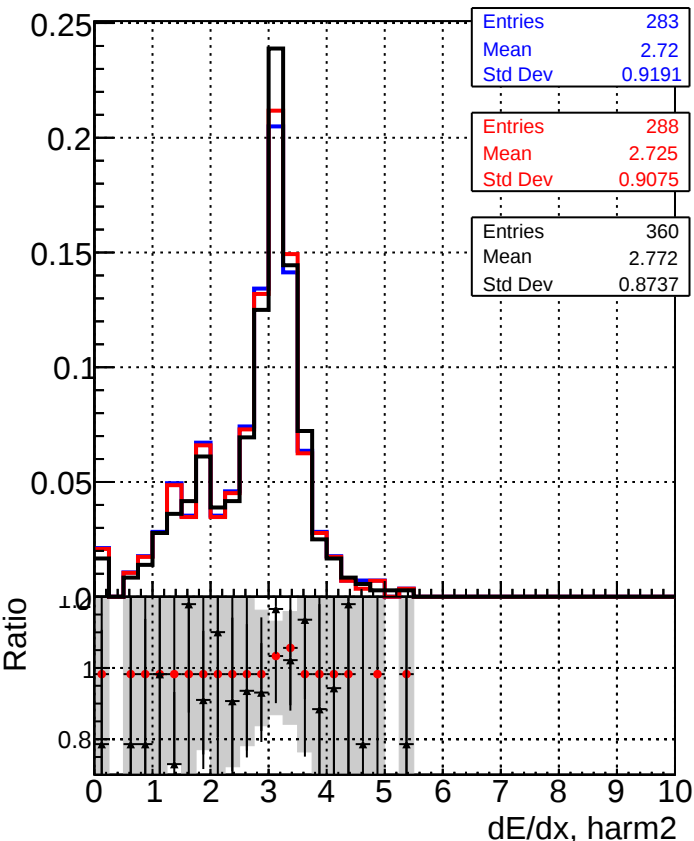
— DQM_CKF-test_1000evt — DQM_CKFREFit-test_1000evt — DQM_mkFitREFit-test_1000evt
