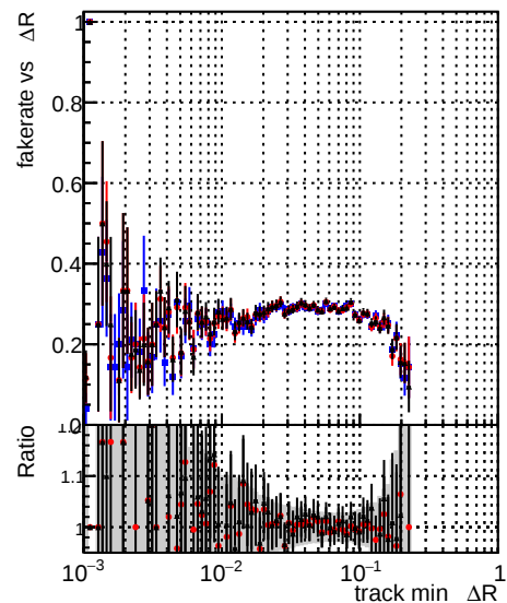
DOM_CKF-test_1000evt DOM_CKFREFit-test_1000evt DOM_mkFitREFit-test_1000evt
