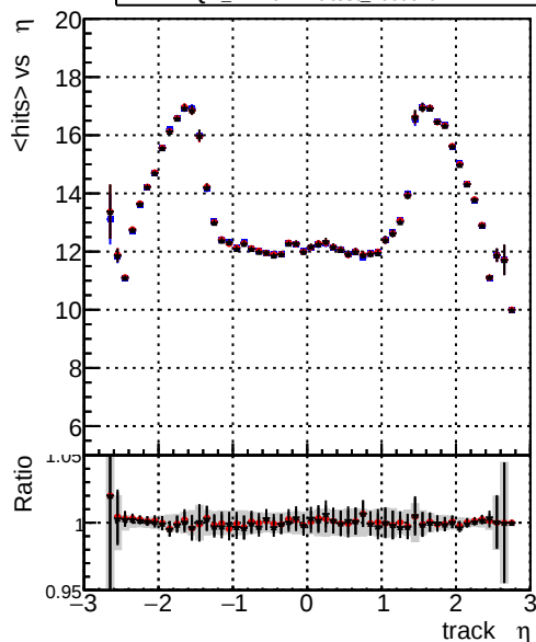
mean hits vs \eta — DQM_CKF-test_1000evt — DQM_CKFFit-test_1000evt — DQM_mkFitREFit-test_1000evt
