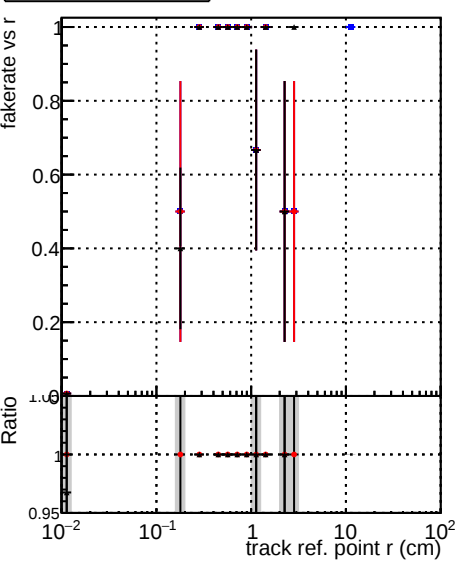
Fake rate vs DOM_CKF-test_1000evt DOM_CKFREFit-test_1000evt DOM_mkFitREFit-test_1000evt
