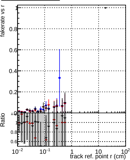
Fake rate vs verpos DOM_CKF-test_1000evt DOM_CKFREFit-test_1000evt DOM_mkFitREFit-test_1000evt
