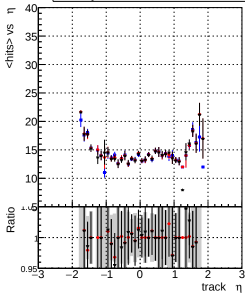
mean hits vs \eta DQM_CKF-test_1000evt DQM_CKFREFit-test_1000evt DQM_mkFitREFit-test_1000evt
